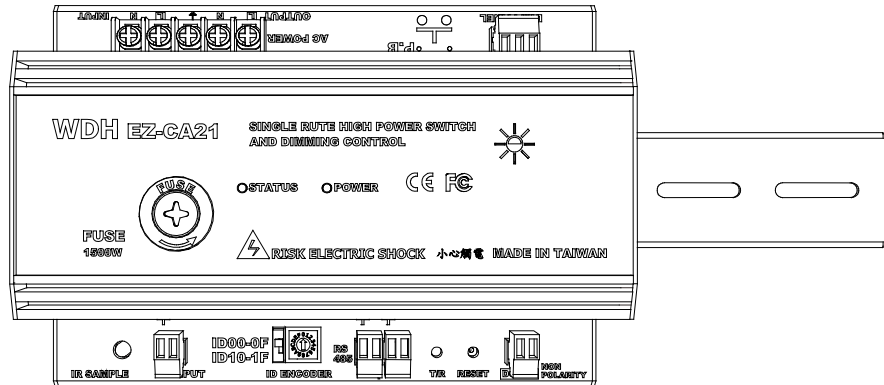
EZ-CA21 可整合標準鋁軌
