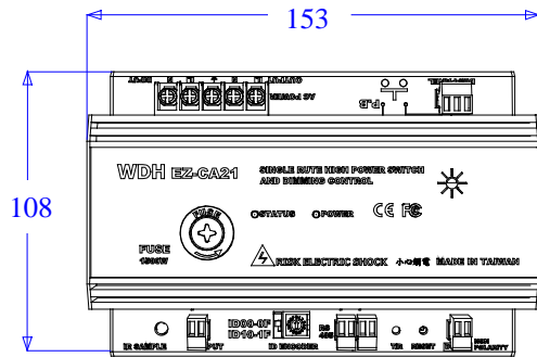
EZ-CA21 頂視圖
